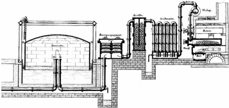
Gasfabriek, schema fabricage steenkoolgas in1860
