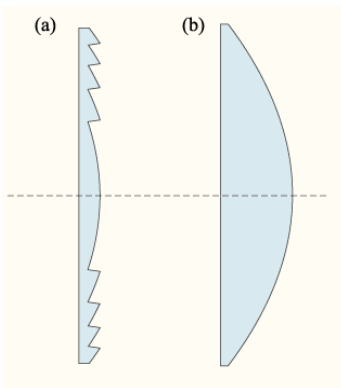
A: doorsnede Fresnel-lens b: doorsnede gewone lens
