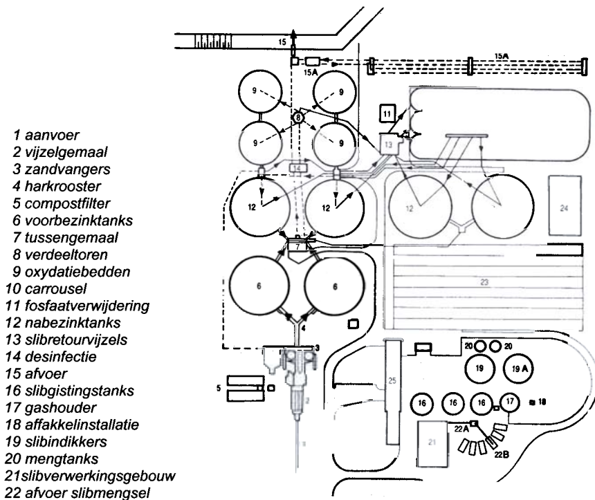
Schema rioolwaterzuiveringsinstallatie Harderwijk
